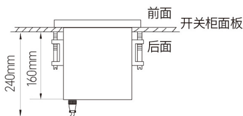
安装示意图
