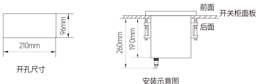
HKJK-3F 智能监控装置安装尺寸及安装示意图
